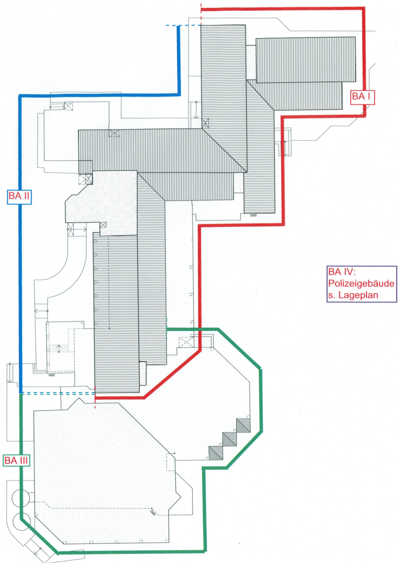
Bauabschnittsplan BA I-III o.M.
