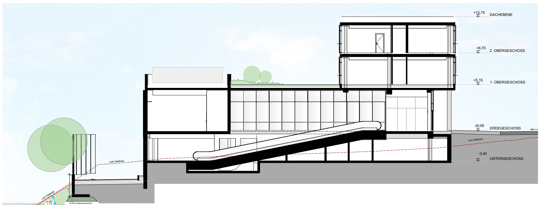
SNITT FAHRSTEIGE
