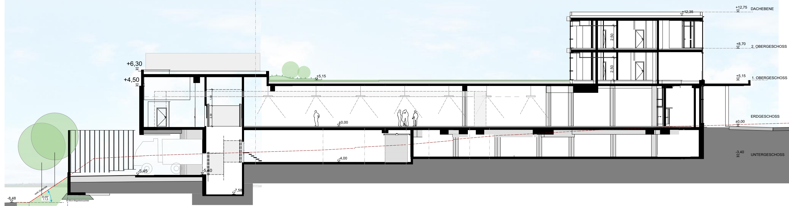
SNITT ANLIEFERUNG
