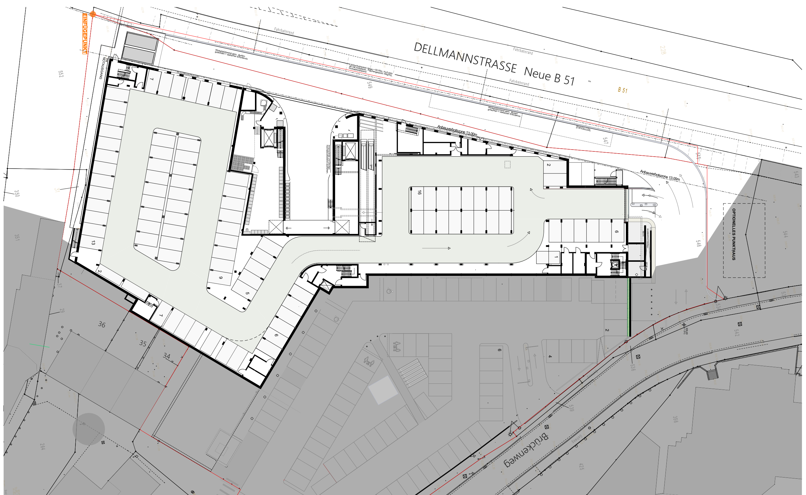
UNTERGESCHOSS
